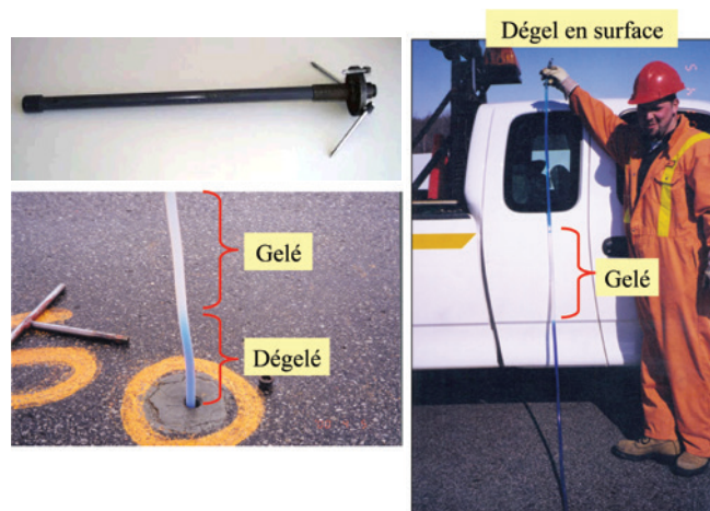
Figure 1: Gelmètre – Lecture d'un gelmètre
