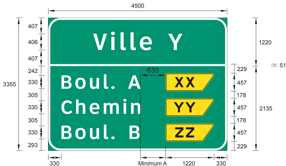
Figure 4.3-7 Exemple de panneau de signalisation d'une suite d'échangeurs rapprochés avec des écussons de sortie
