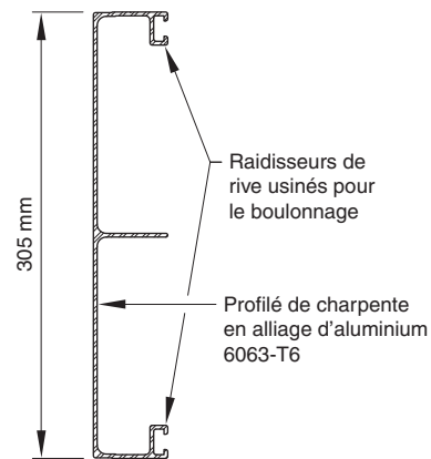
Figure 1.2-1 Vue de côté d'un profilé
