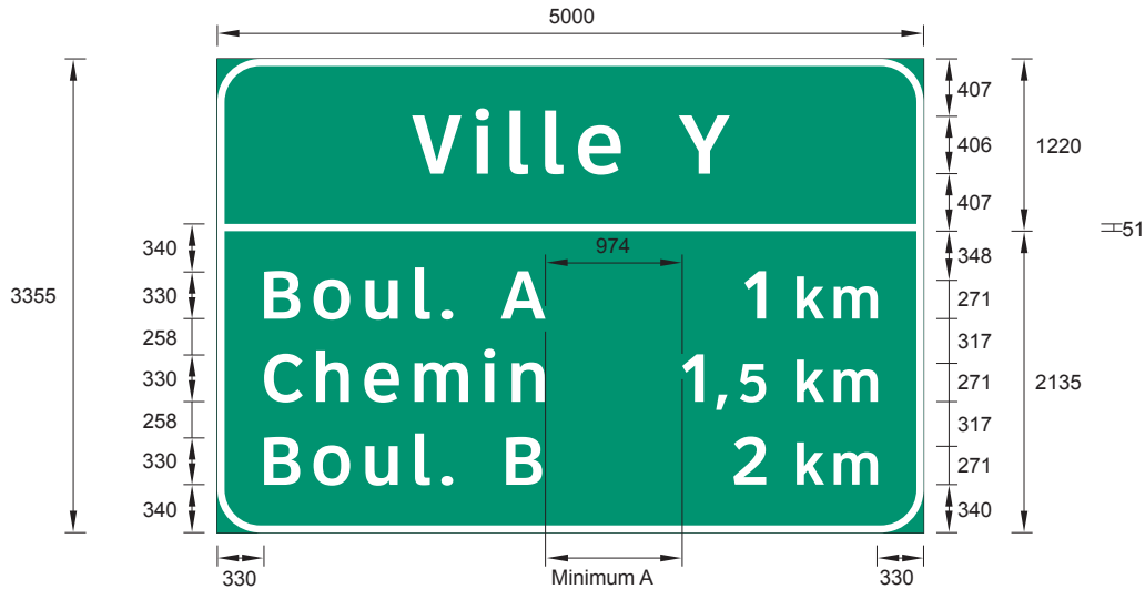
Figure 4.3-6 Exemple de panneau de signalisation d'une suite d'échangeurs rapprochés à l'entrée d'une agglomération (I-70-2)
