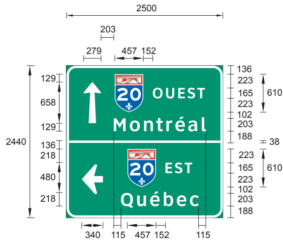
Figure 4.5-2 Exemple de panneau d'accès à l'autoroute (I-90)
