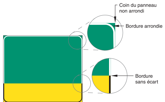
Figure 1.2-3 Vue d'un coin et d'une bordure de panneau ayant deux sections
