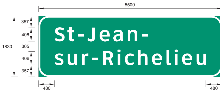
Figure 4.3–3 Exemple de panneau d'entrée d'agglomération (I-150-4)
