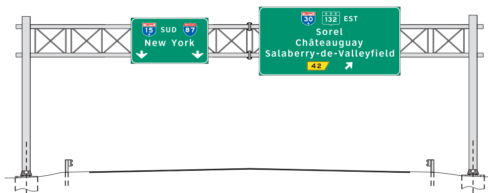
Figure A.1-3 Exemple de calcul du nombre d'unités de mots pour un panneau installé sur un portique
