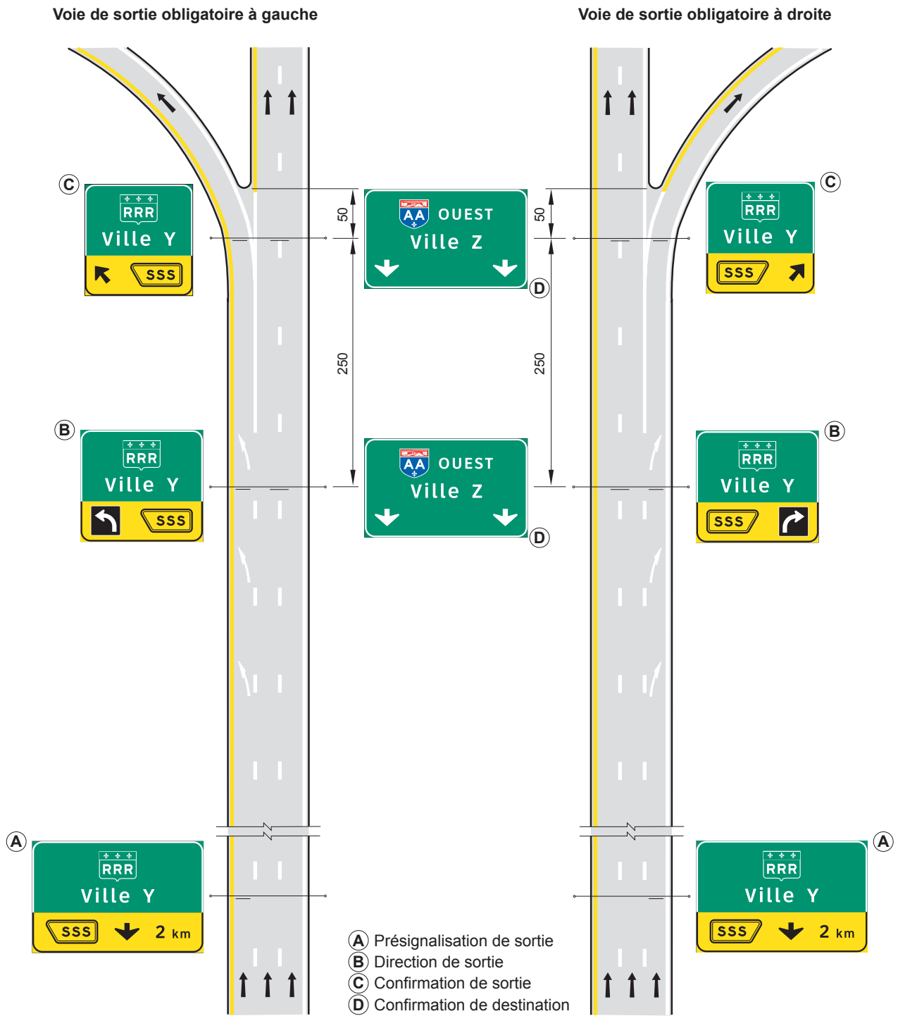
Figure 4.2-1 Exemples de séquence de panneaux dans une voie de sortie obligatoire
