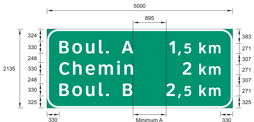
Figure 4.3-5 Exemple de panneau de signalisation d'une suite d'échangeurs rapprochés (I-70-1)
