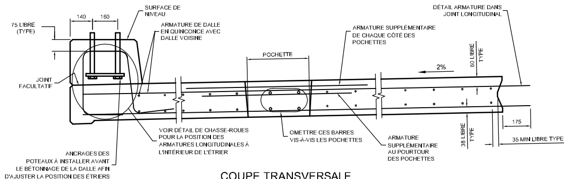
COUPE TRANSVERSALE NON À L'ÉCHELLE
