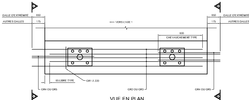
VUE EN PLAN NON À L'ÉCHELLE
