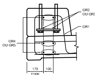
COUPE B-B
