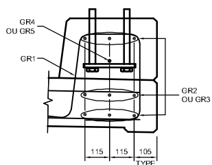
COUPE A-A
