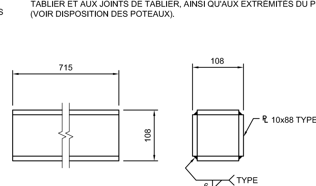
PIÈCE ④
