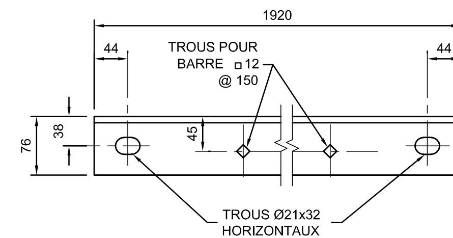
PIÈCE ⑦
