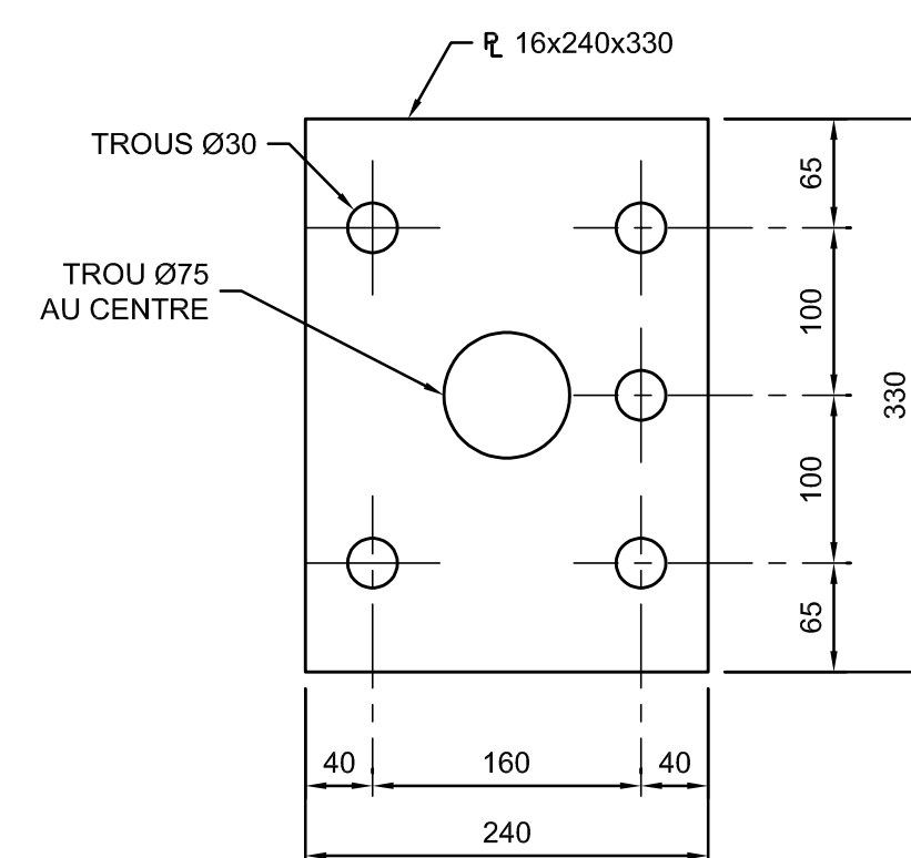
PLAQUE D'ANCRAGE
