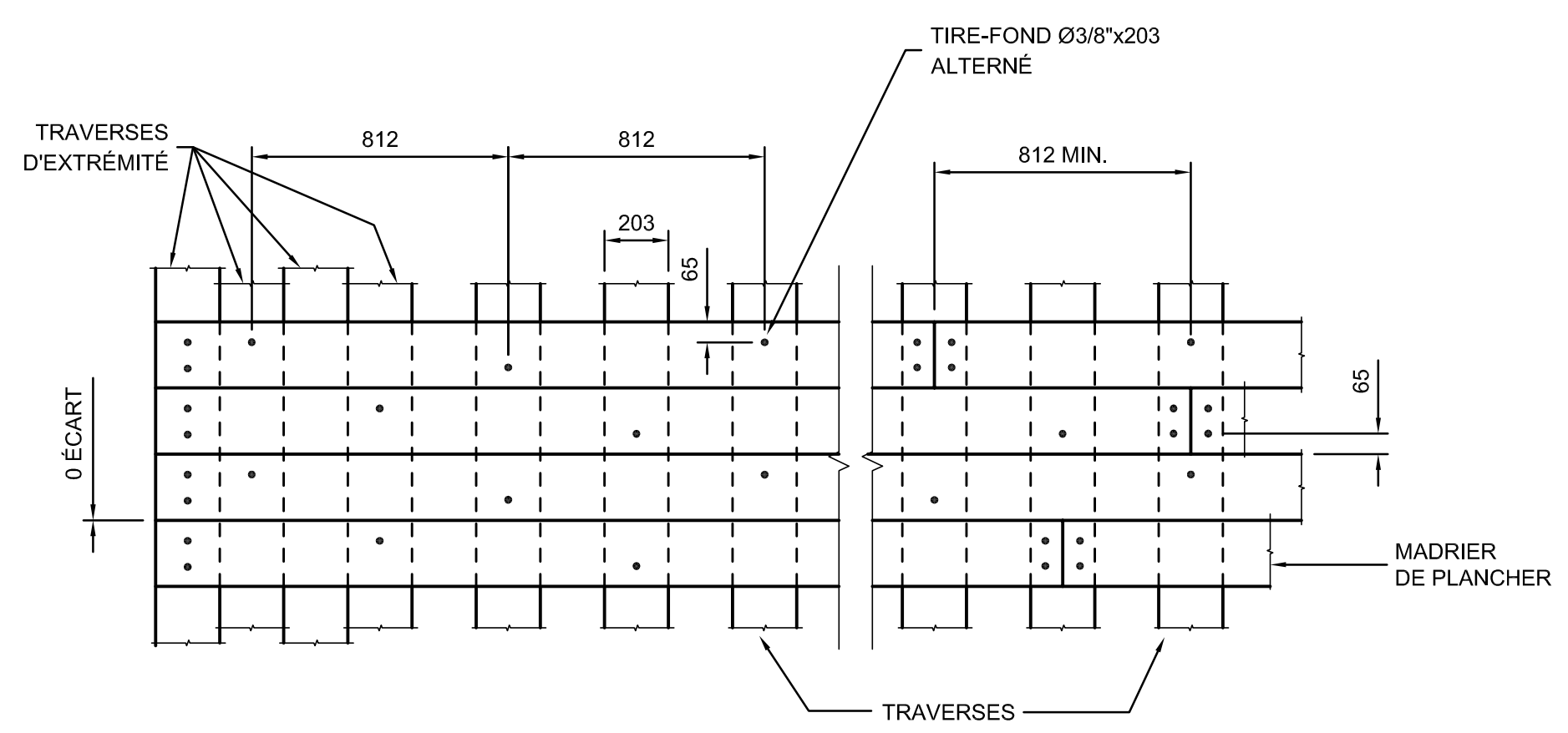
PLAN FIXATION NON À L'ÉCHELLE
