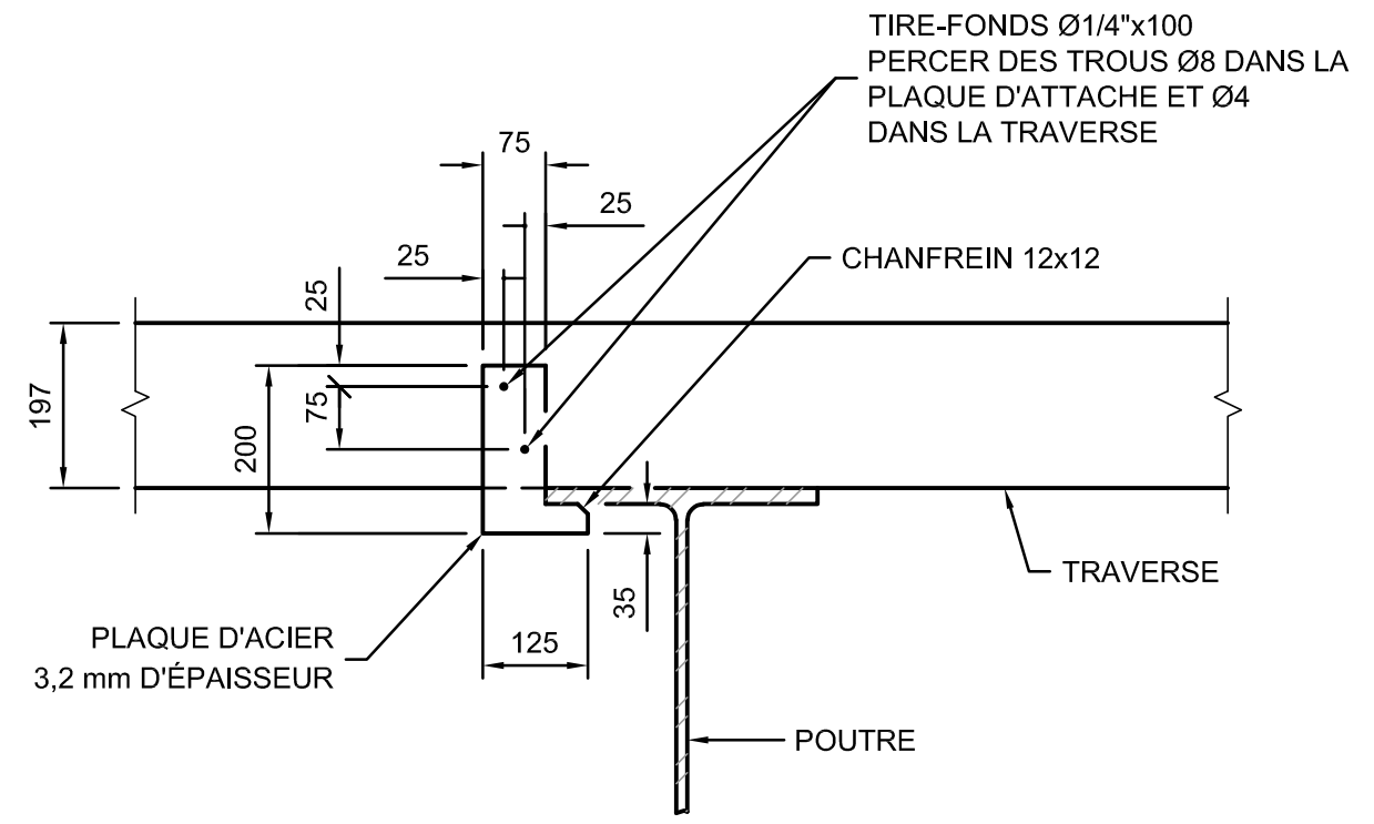
PLAQUE D'ATTACHE NON À L'ÉCHELLE
