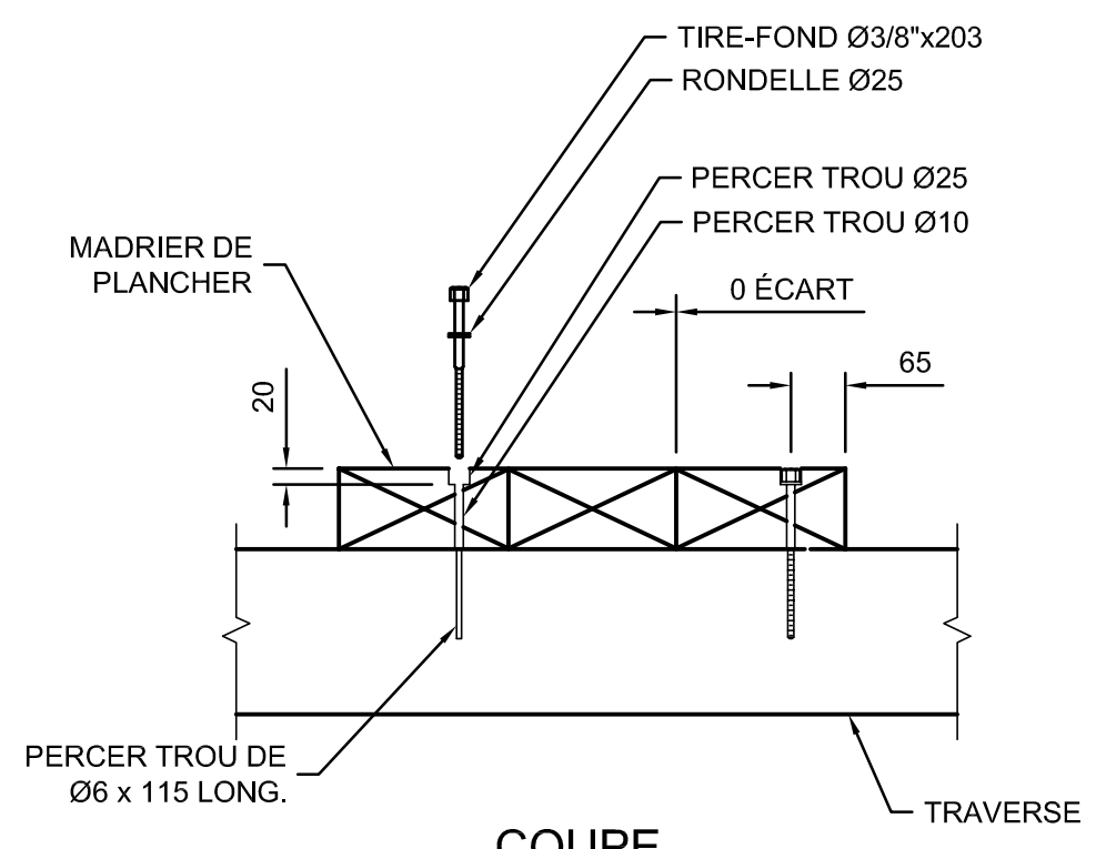
COUPE
