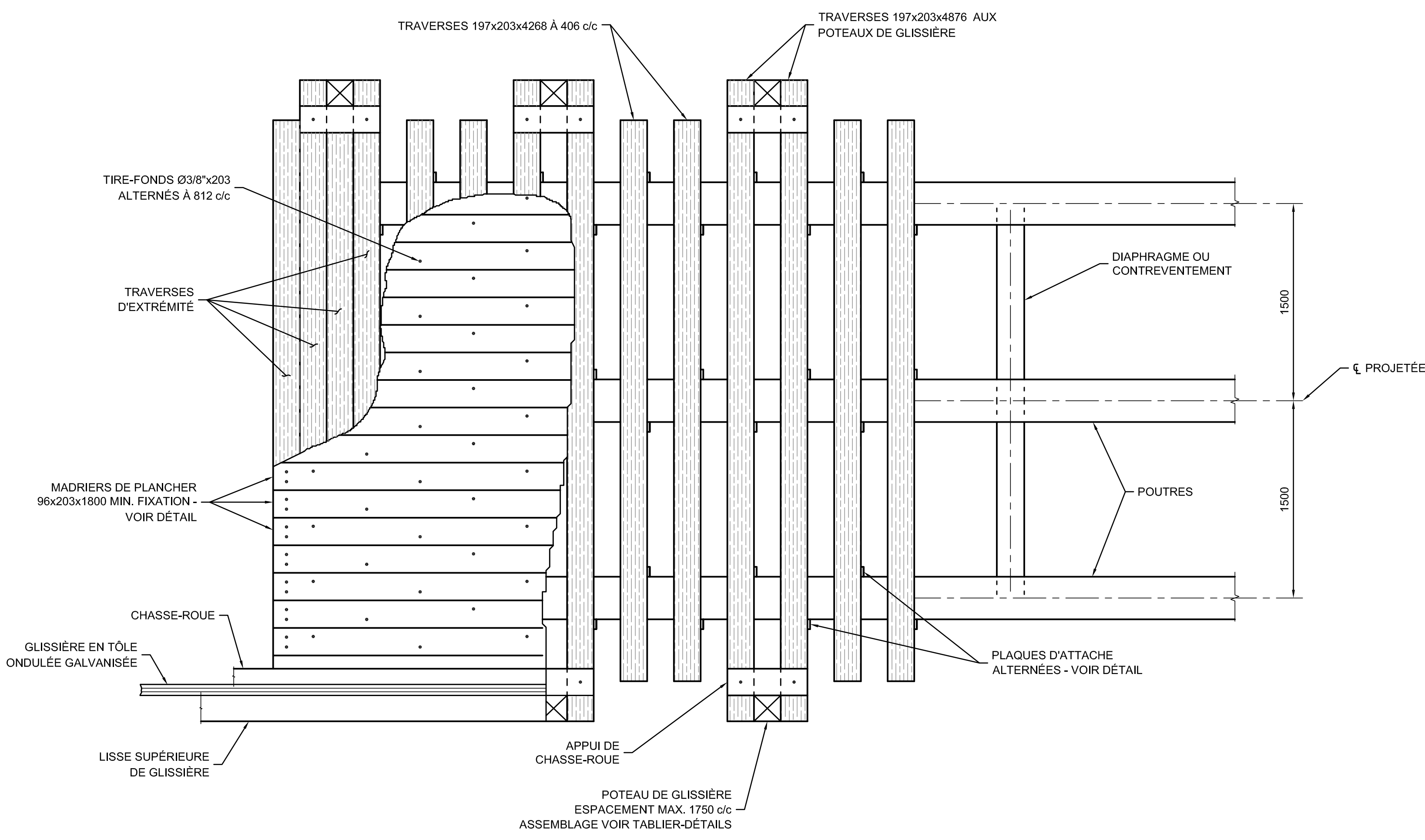
PLAN PARTIEL - PLATELAGE NON À L'ÉCHELLE
