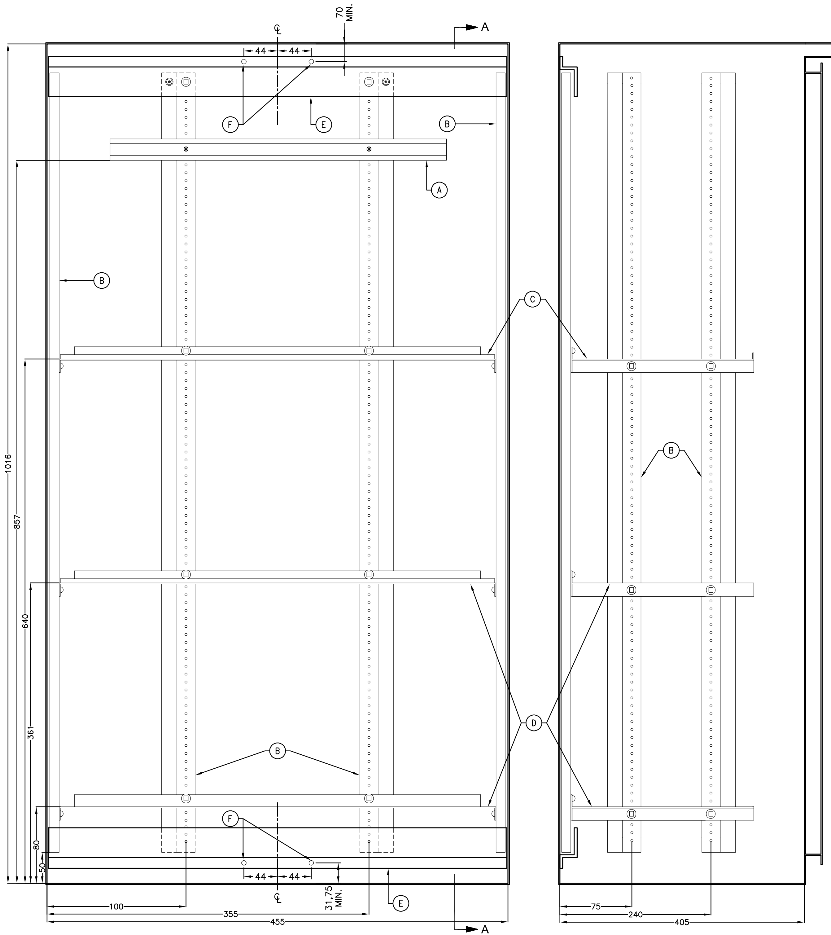
COUPE A-A'
