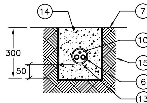
CÂBLES DANS LE ROC
