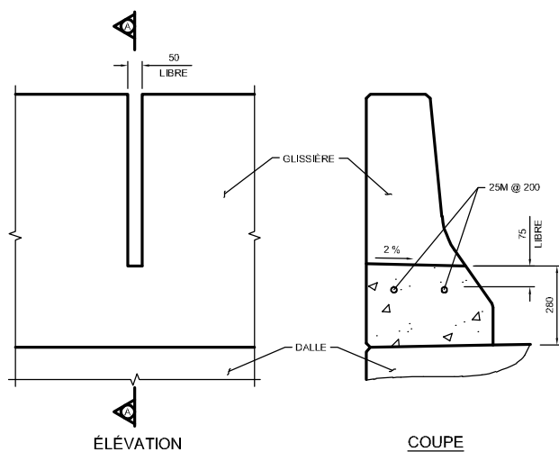
ÉLEVATION
