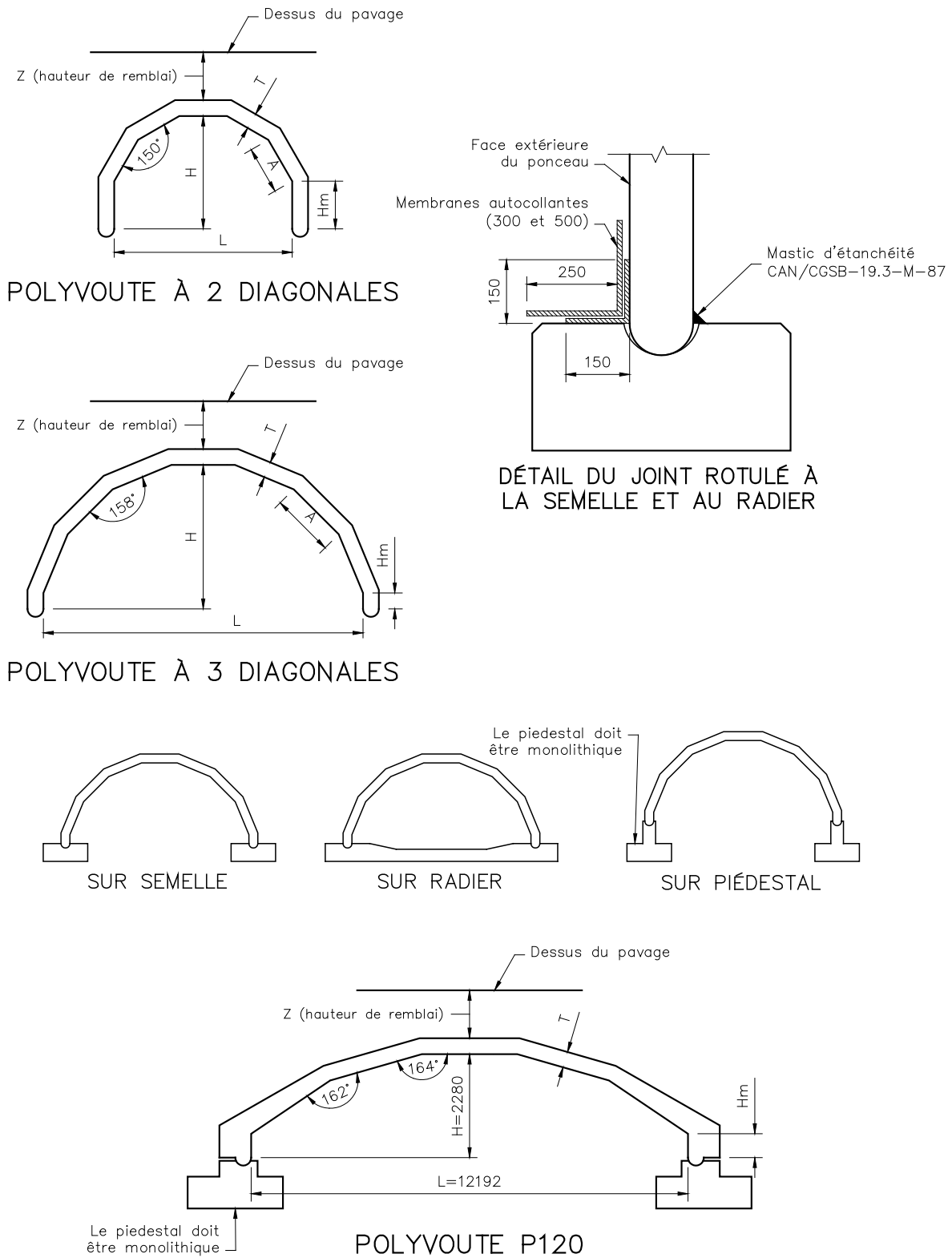
Figure 1 – Détails ponceau POLYVOÛTE
