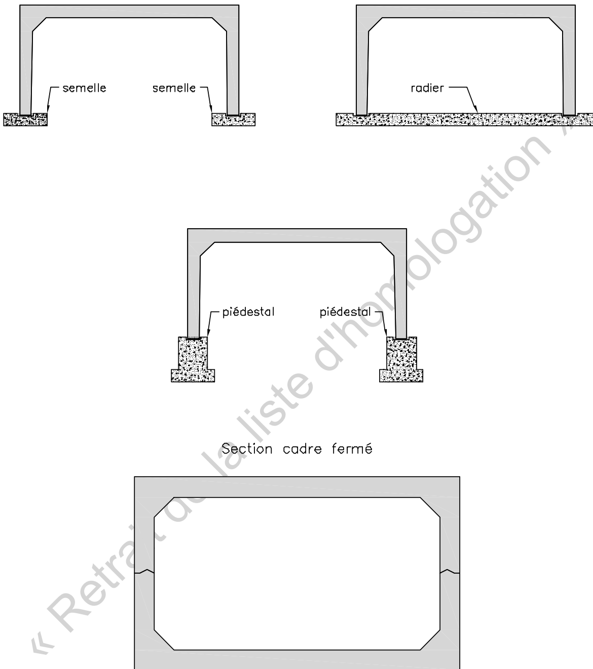
Figure 1 – Géométrie et options de fondations
