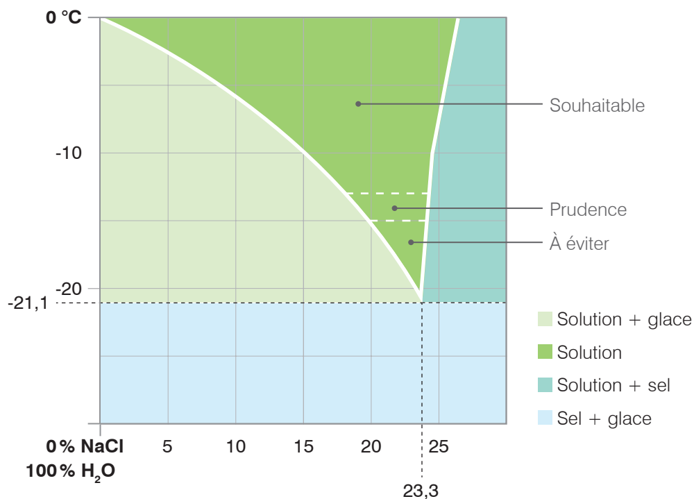
Figure B.1 – Diagramme des phases d'une solution d'eau et de chlorure de sodium
